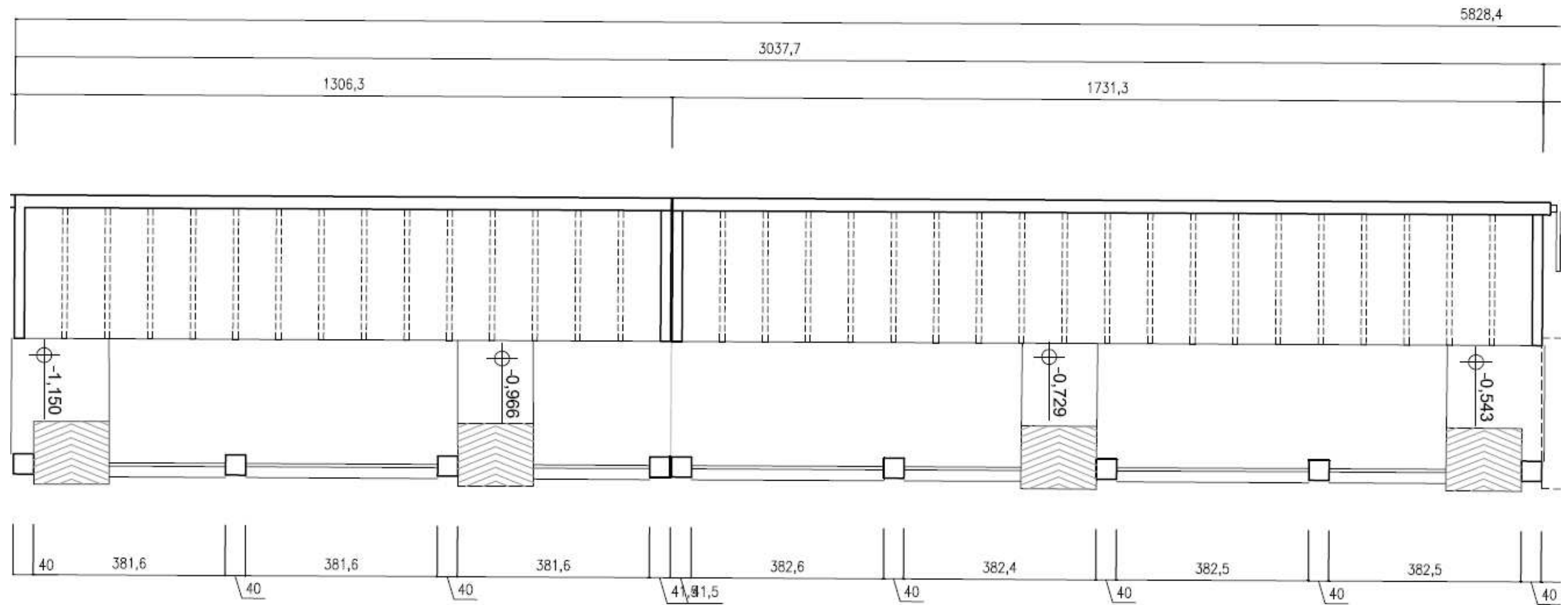
Sezione tipo di un blocco di loculi fuori scala
