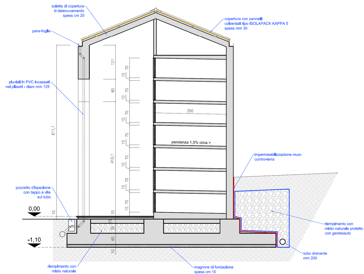
Sezione tipo di un blocco di loculi fuori scala
