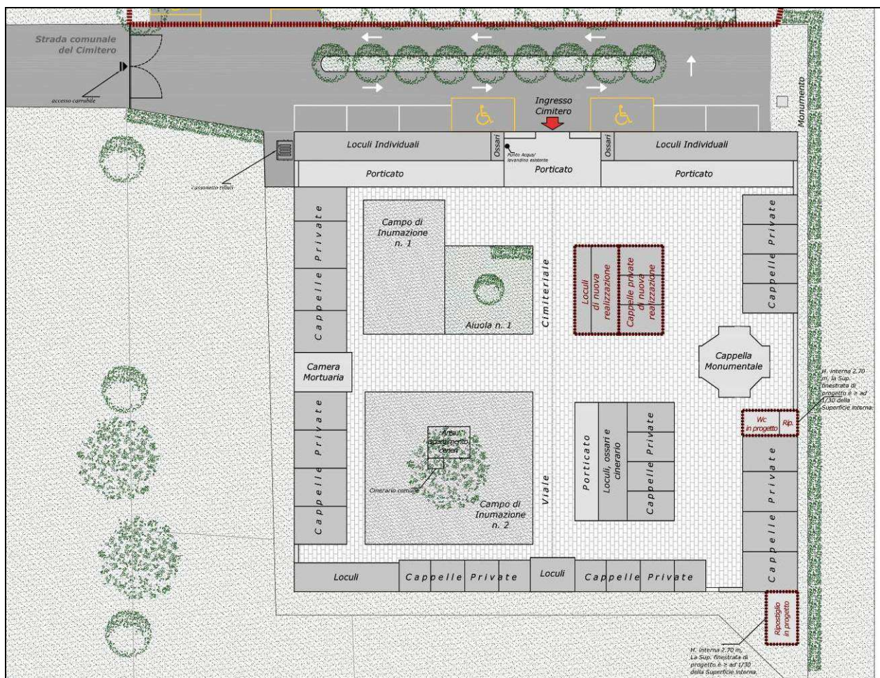
Stralcio planimetrico del progetto di adeguamento del cimitero esistente fuori scala
